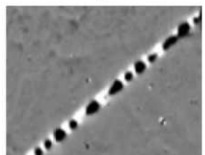
Wasserleitungsrohr aus Eisen (Dynamik +/-50 nT), Bildbreite 30 m
